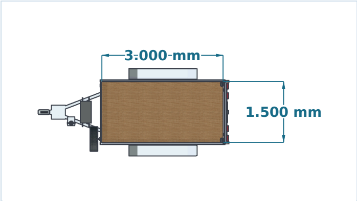
Bovenaanzicht met maten
