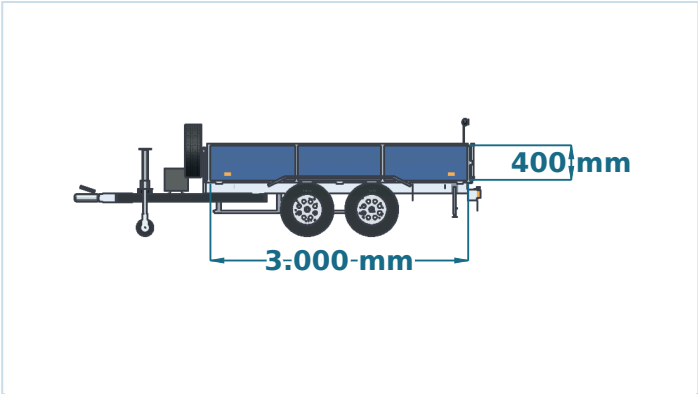
Zijaanzicht met maten
